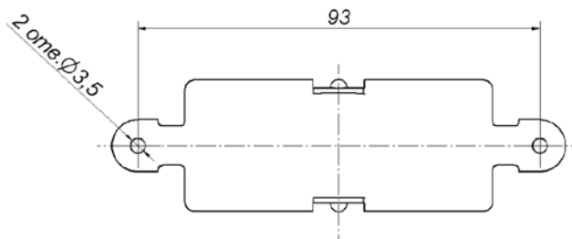
Рисунок 2 – Расположение отверстий для крепления извещателя.
